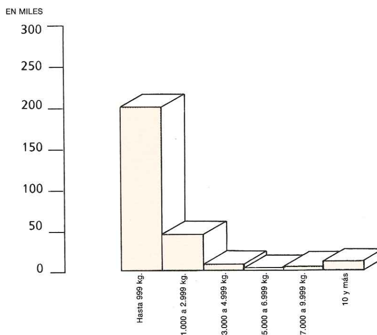
DISTRIBUCION DE CAMIONES SEGUN CARGA
